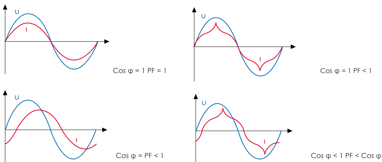
Figur 10: Linjär och olinjär ström
