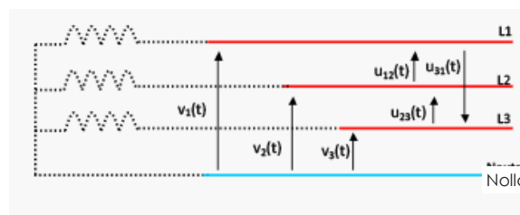
Figur 3: 3-fas distributionssystem.
