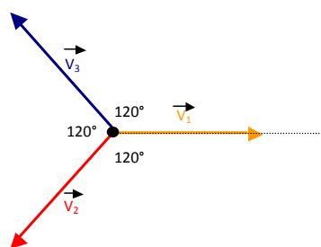
Figur 7: Ett trefassystems vektordiagram
