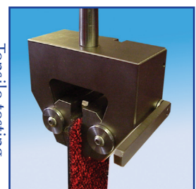
Tensile testing
